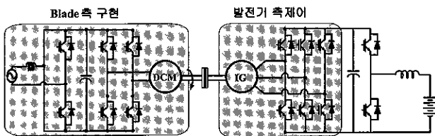
그림 3 터빈시뮬레이터 구성도 Fig 3 Turbine simulator
