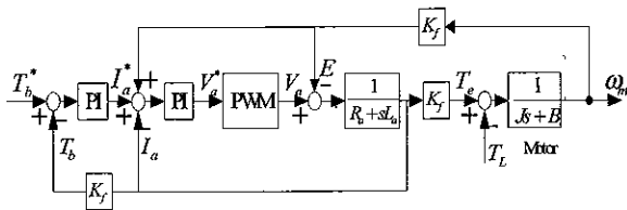
그림 4 직류전동기 제어 블럭도 Fig 4 Block diagram of dc motor control
