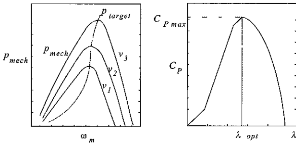
그림 5 풍력터빈의 출력 특성 (a) 회전속도에 대한 출력전력 (b) 주속비에 대한 전력변환계수 Fig 5 Output characteristics of wind blade (a) output power versus rotational speed (b) power conversion coefficient versus blade tip-speed ratio
