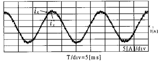
그림 14 전원전류 제어
