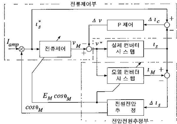
그림 5 전원전류제어 블록도
