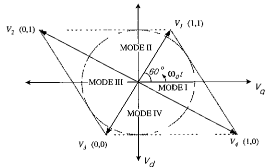
그림 8 2-leg 인버터의 공간전압벡터도 Fig 8 Space voltage vector diagram for 2-leg inverter
