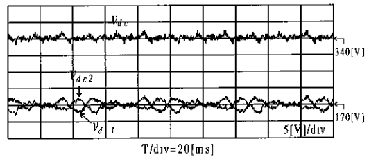
그림 16 직류전압 제어
