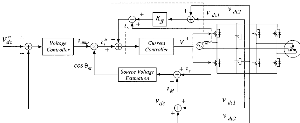
그림 6 단상 반파 PWM 정류기의 전체 제어블록도 Fig 6 Overall control block diagram of single-phase half-bridge PWM converter
