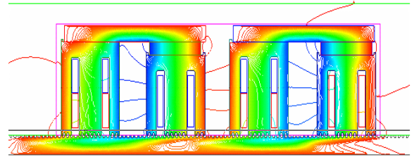
그림 1 LHSM의 자속 분포 Fig. 1 PM flux lines in LHSM
