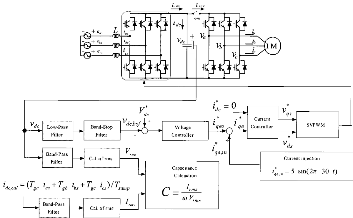
그림 1 직류 커패시터를 추정하기 위한 제어 블록도 Fig 1 Control block diagram of 3-phase PWM converter for estimating dc capacitance
