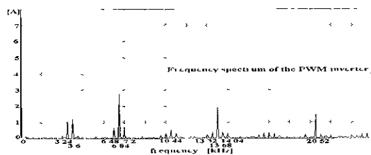
(b) PWM 인버터 입력 측 직류링크 전류(60Hz) (b) Dc link current of PWM inverter input side(60Hz)
