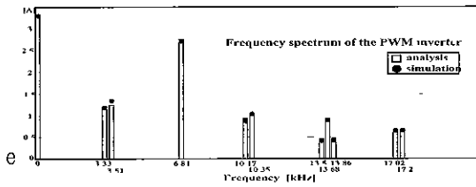
(b) PWM 인버터 입력측 직류링크 전류(20Hz) (b) Dc Link current of PWM inverter input side
