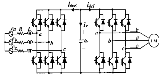
그림 1 3상 ac/dc/ac PWM 컨버터 Fig 1 Three-phase ac/dc/ac PWM converter
