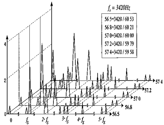
그림 12 비동기 PWM의 경우 커패시터 전류의 고조파 스펙트럼 Fig 12 Harmonic spectrum of dc capacitor current for asynchronous PWM
