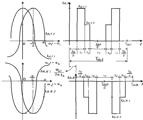
그림 5 상전류와 직류링크 전류와의 관계 (위) 인버터 측 (아래) 컨버터 측 Fig 5 Relation of phase current and dc link current (top) inverter (bottom) converter
