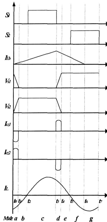
그림 4 정상상태 시의 각부의 이론 파형 Fig. 4 Main theoretical waveforms in steady state
