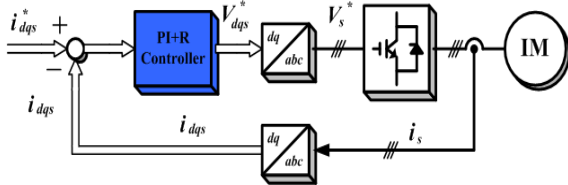
그림 8 PI + Resonant 전류제어기 블록도 Fig. 8 Block diagram of PI+resonant current controller
