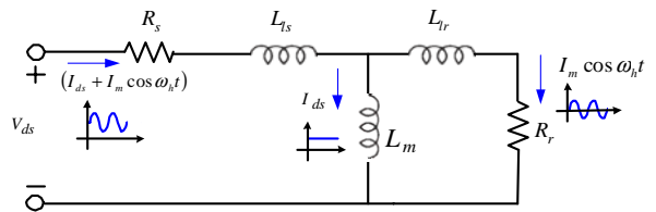
그림 2 정지 상태에서의 유도전동기 d축 등가회로 Fig. 2 D-axis equivalent circuit of an IM at standstill
