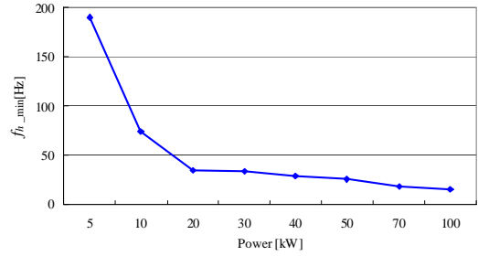
그림 4 고주파 전류시험을 위한 용량별 최소주입주파수 Fig. 4 Plot of f_{h\_min} on commercial IMs for HF current test
