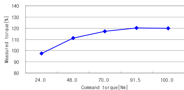
그림 15 IM#3의 추정된 상수를 이용한 부하토크 실험결과 Fig. 15 Load torque test results for estimated parameters of IM#3
