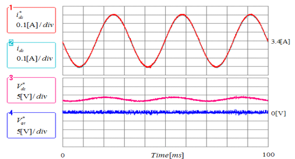
그림 11 30[Hz] 저주파전류제어 성능 Fig. 11 LF current control performance at 30 Hz
