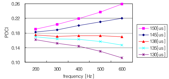
그림 7 IM #1 구동장치의 PDCI ( K_\delta ) 측정 결과
